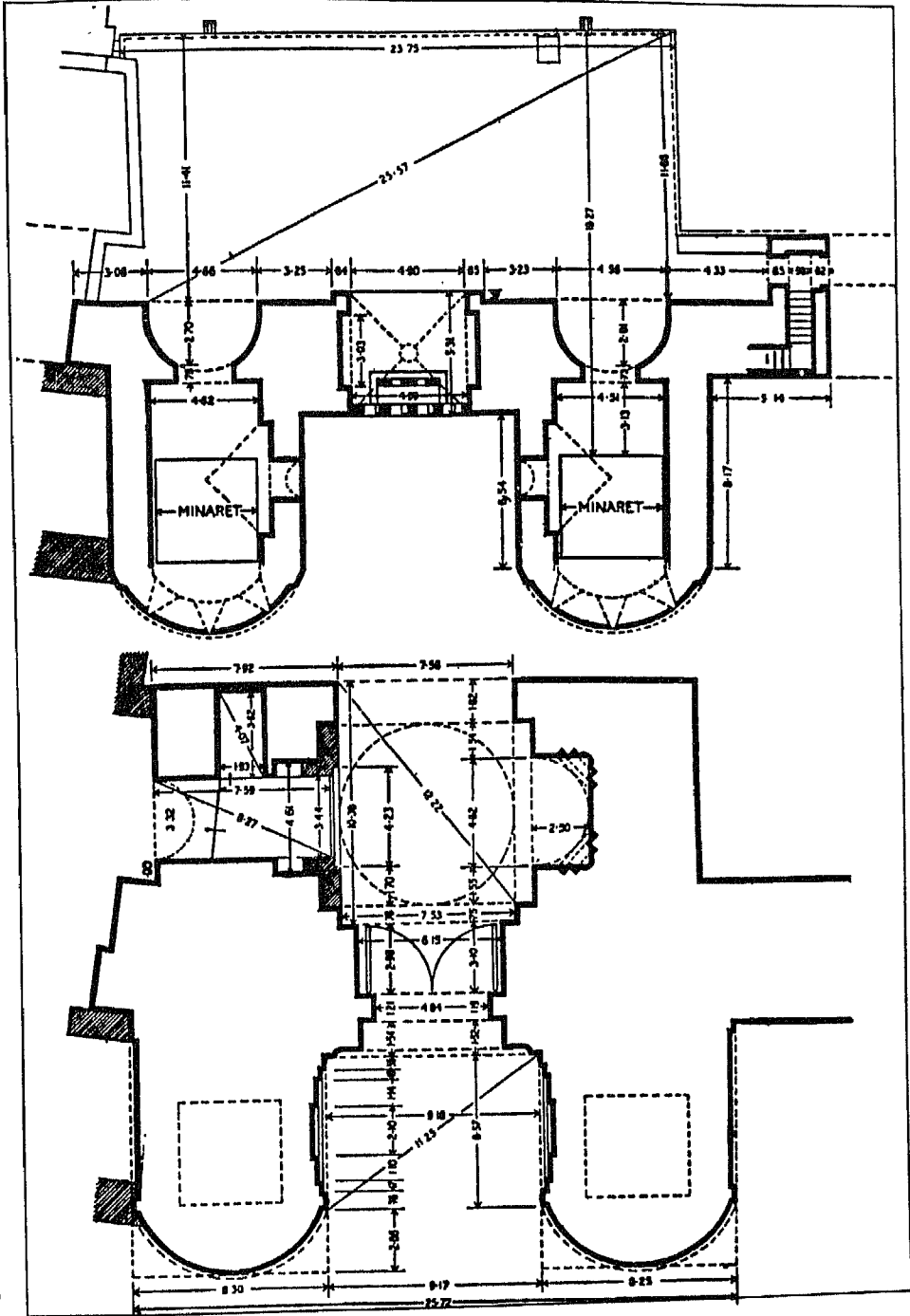
شكل (١٣) باب زويلة، مسقط أفقي، عن كريزويل
